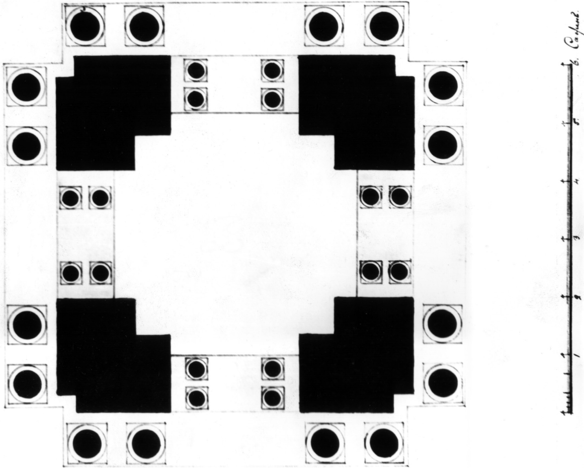
План 2-го яруса колокольни (проект Е. А. Васильева).
