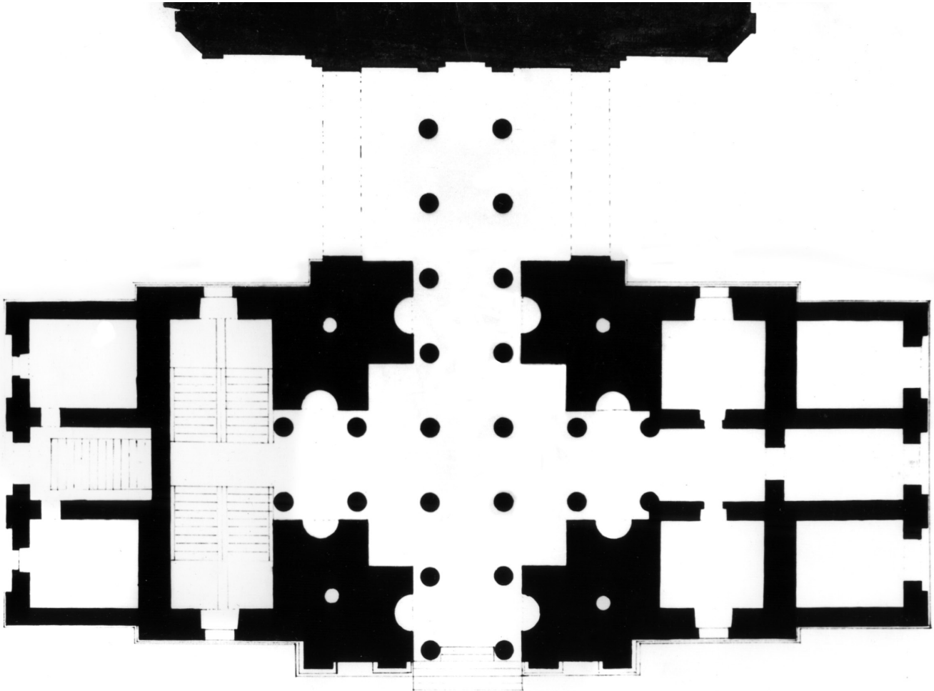
План 1-го яруса колокольни. (проект Е. А. Васильева 1-й вариант).
