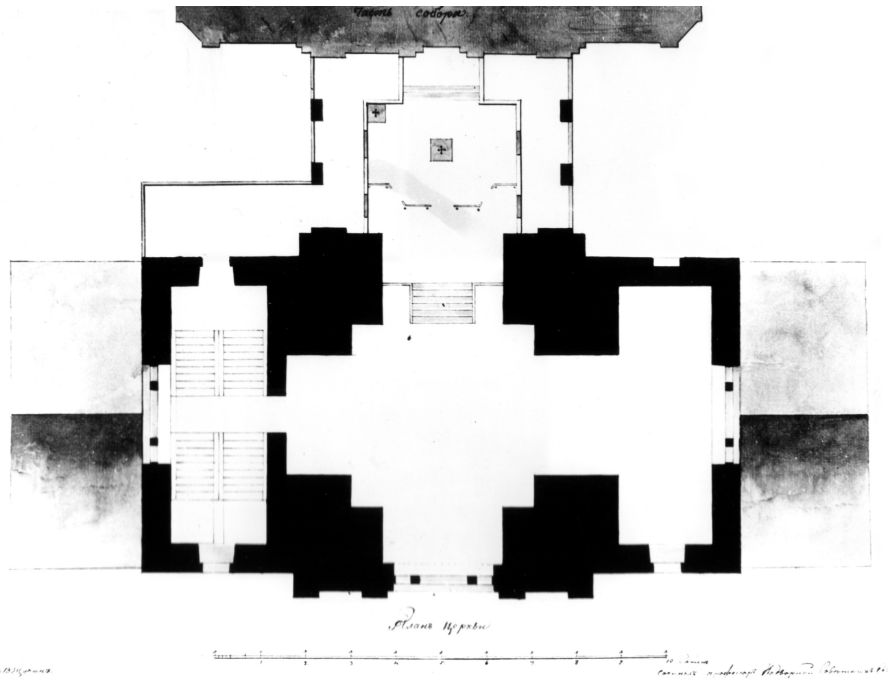
План 2-го этажа 1-го яруса колокольни (проект Е. А. Васильева).
