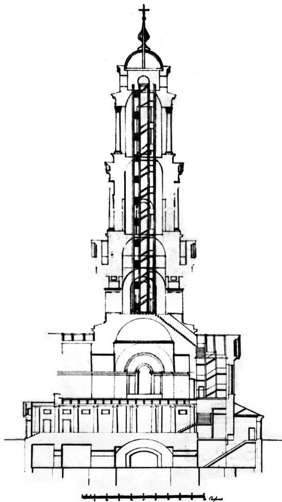
Разрез колокольни Успенского собора (проект Е. А. Васильева).
