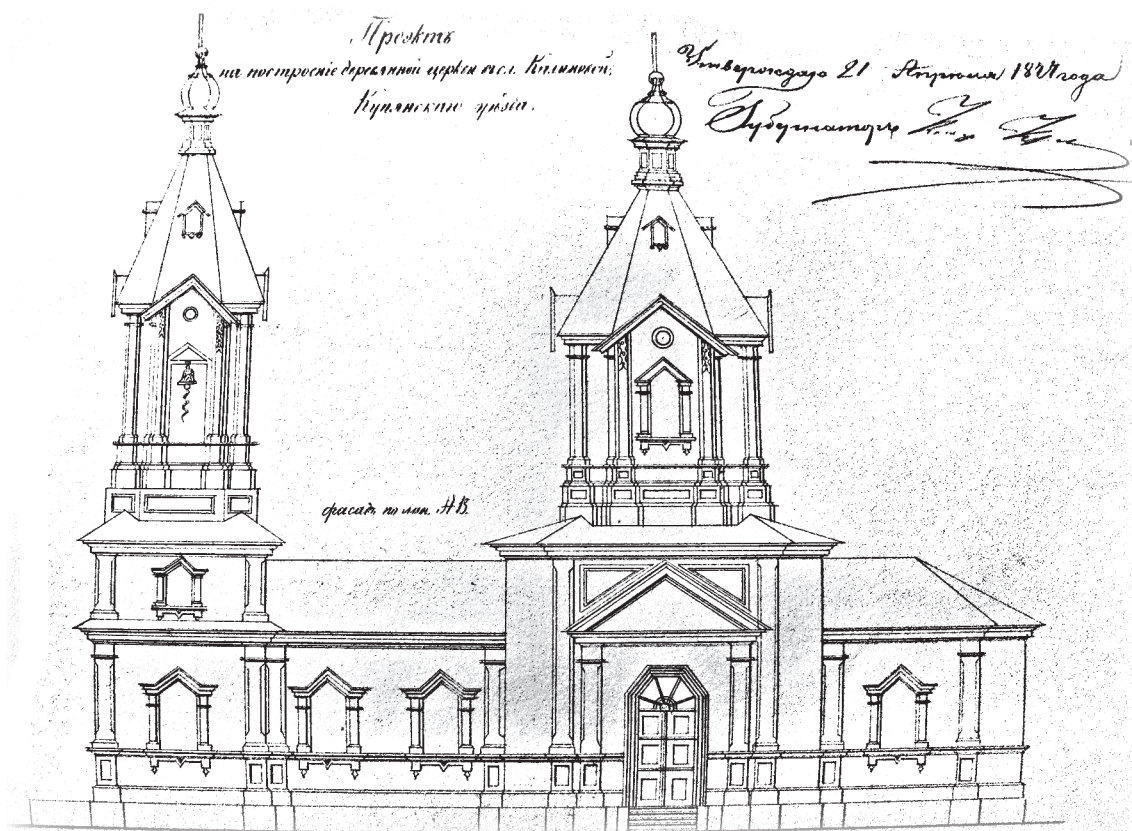
Проект постройки Владимир-Богородицкой церкви в с. Калиновом
