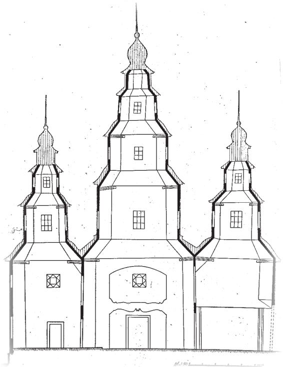
с. Осиновая, Архангело-Михайловская церковь, поперечный разрез
