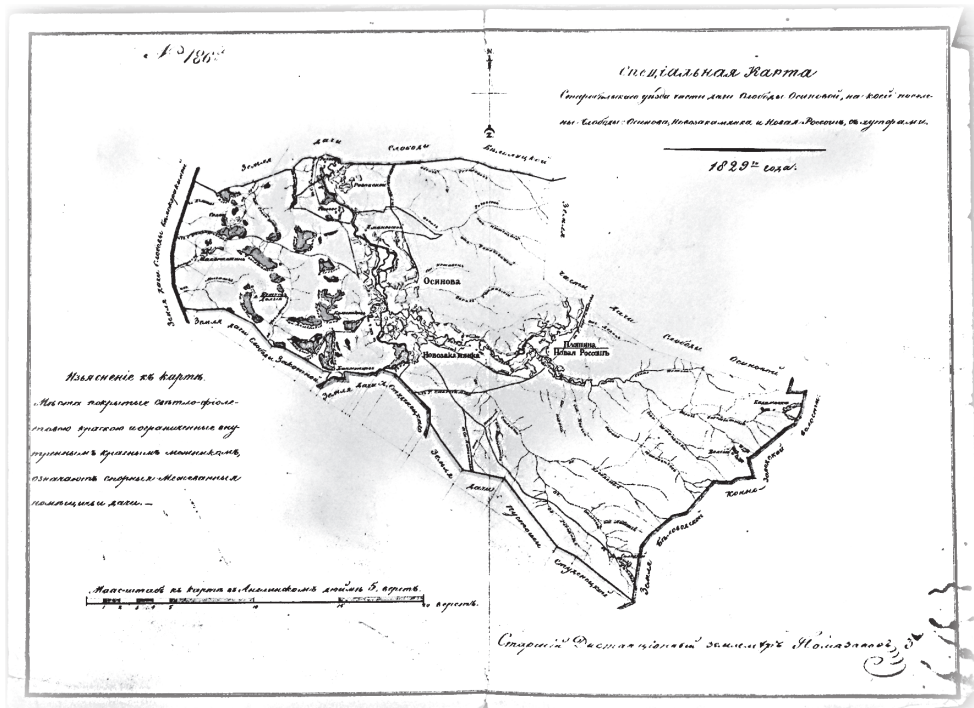
с. Осиновая, топографический план, 1829 г.
