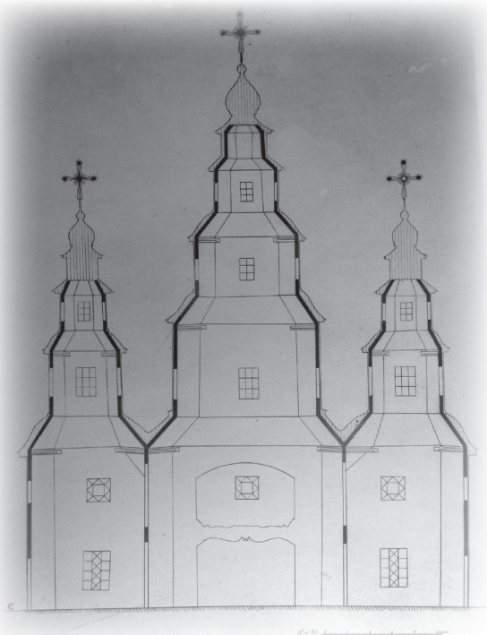
с. Осинава, Архангело-Михайловская церковь, продольный разрез
