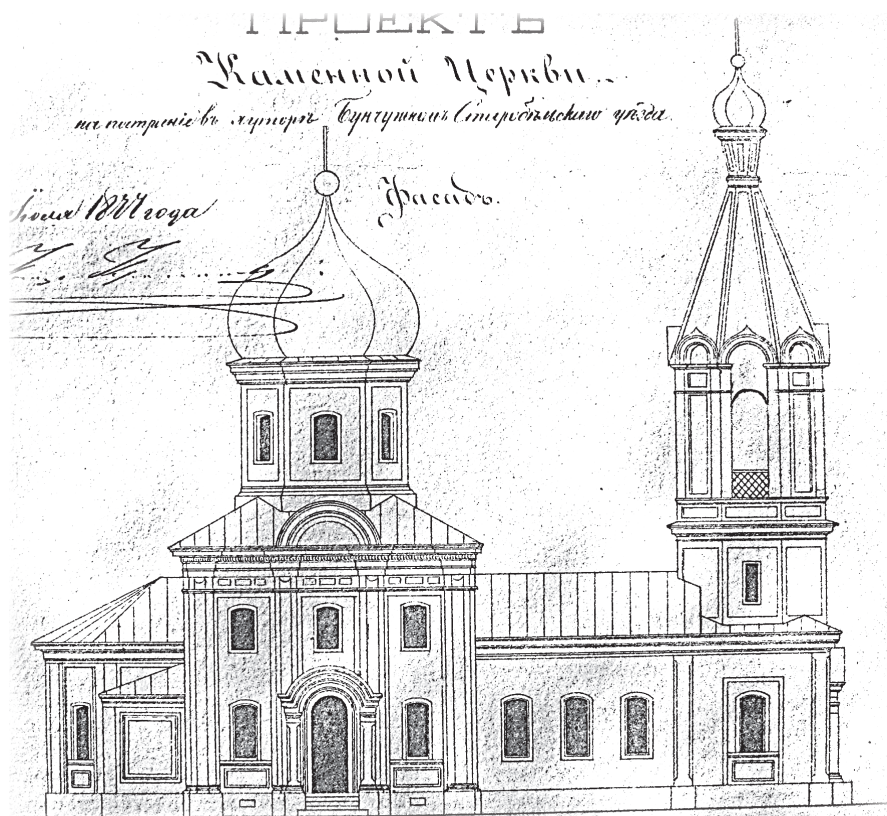
Проект Рождество-Богородицкой церкви в хут. Бунчужном
