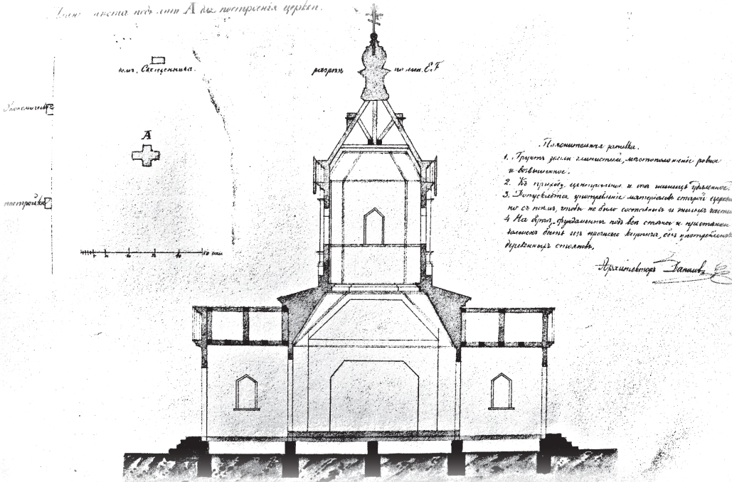
Проект постройки Владимир-Богородицкой церкви в с. Калиновом
