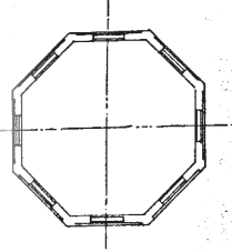
План купола
