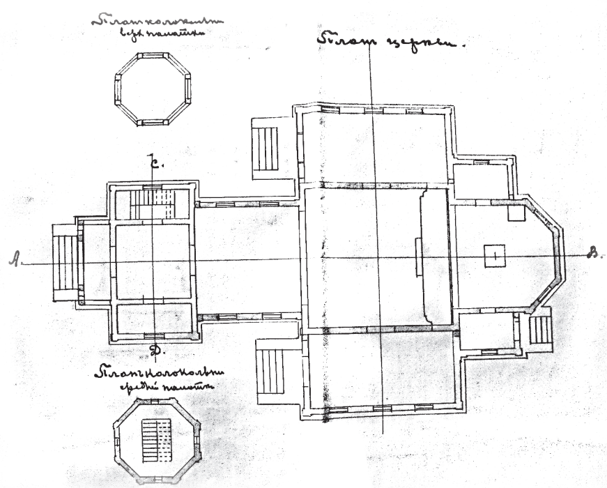
Проект постройки церкви в хут. Овзаров
