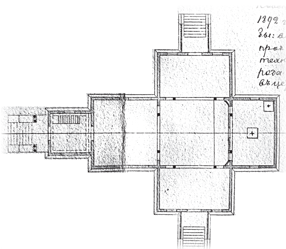
Обмерный чертеж деревянной церкви в с. Голубовка
