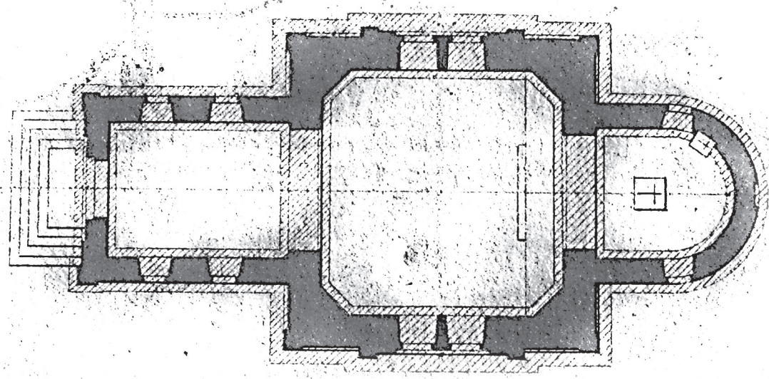
Проект Иоанно-Богословской церкви в хут. Лубянка
