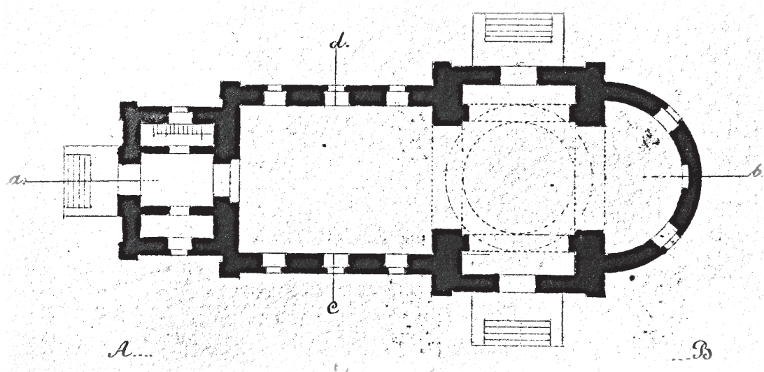
Проект постройки Георгиевской церкви в сл. Ново-Павловка
