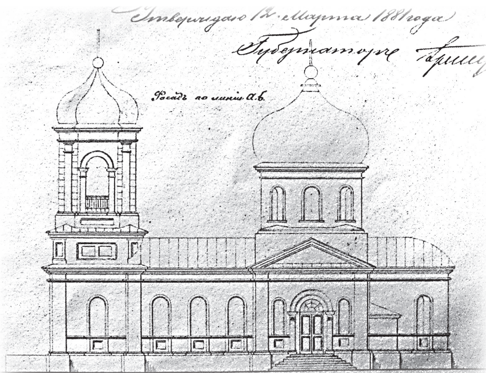
Проект постройки Николаевской церкви в сл. Муратовой
