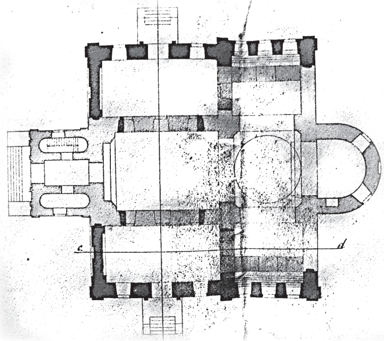
Проект расширения Успенской церкви в сл. Литвиновка
