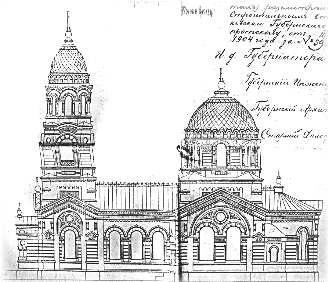
Прект постройки Иоанно-Предтегевской в сл. Меловатка
