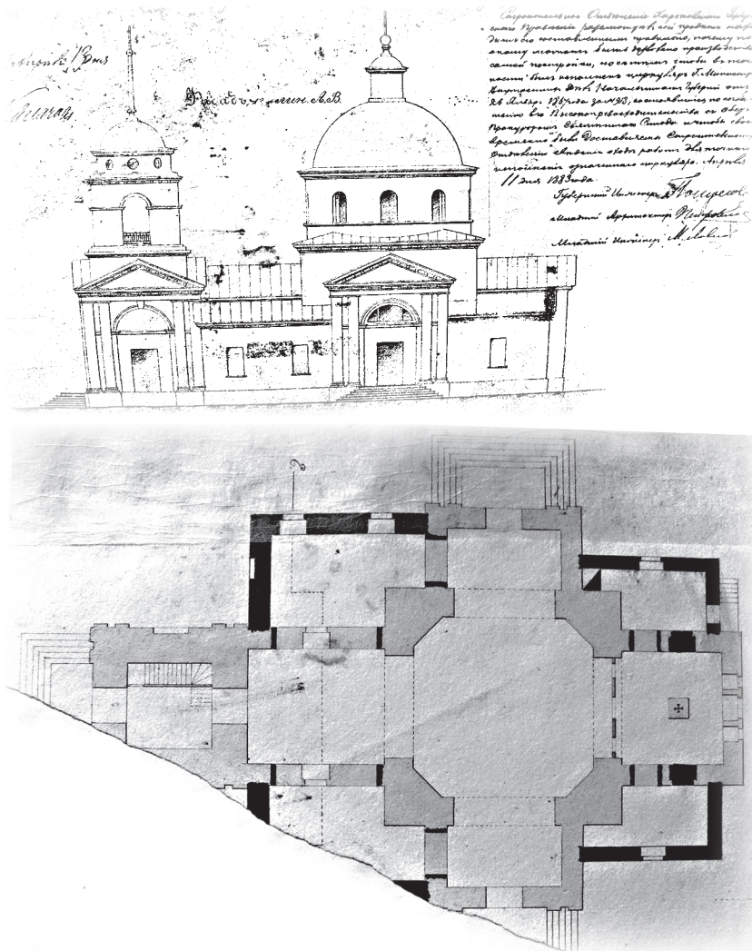
Проект постройки Петропавловской церкви в с. Подгоровка
