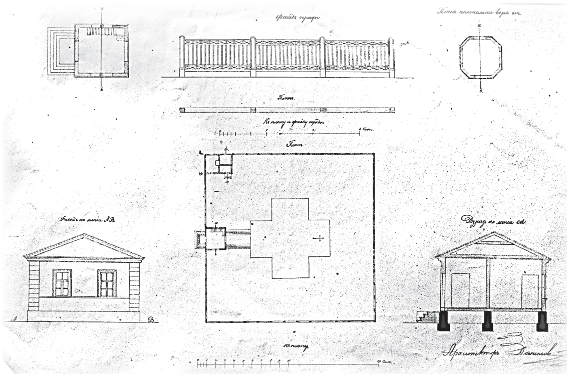
Проект постройки Архангело-Михайловской церкви в с. Воеводское
