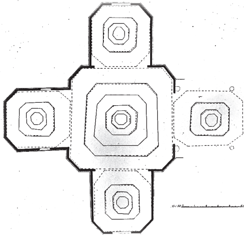
с. Осиновая, Архангело- Михайловская церковь, план
