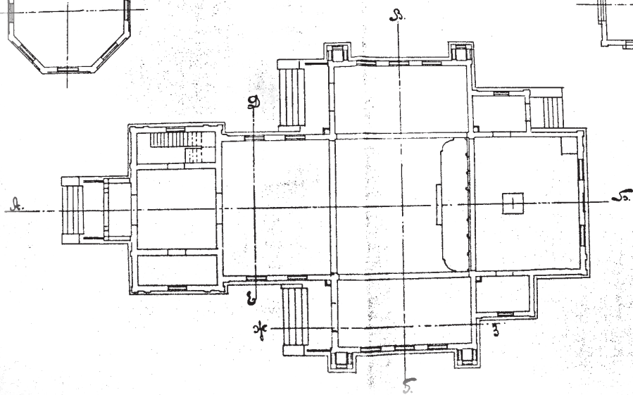
План церкви
