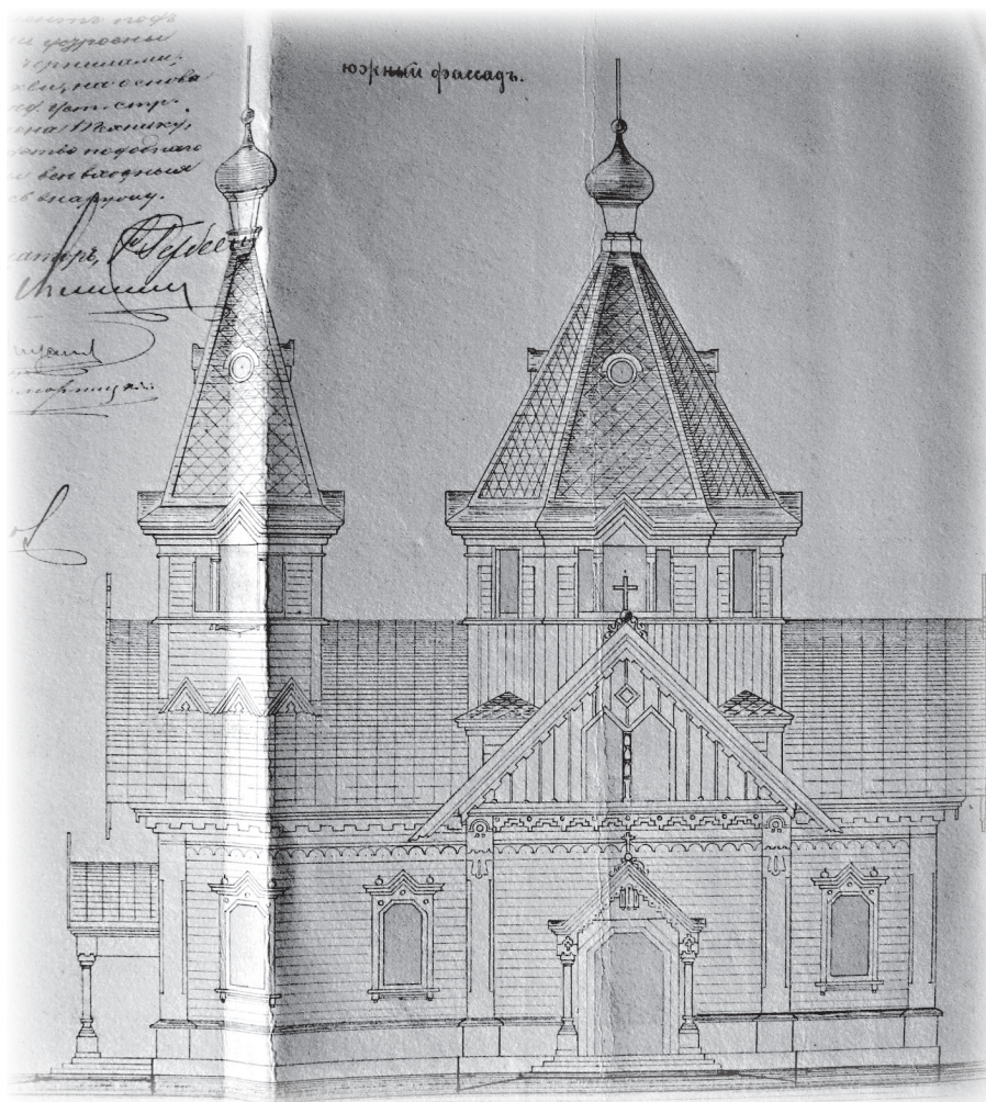
Проект постройки церкви в хут. Павленков
