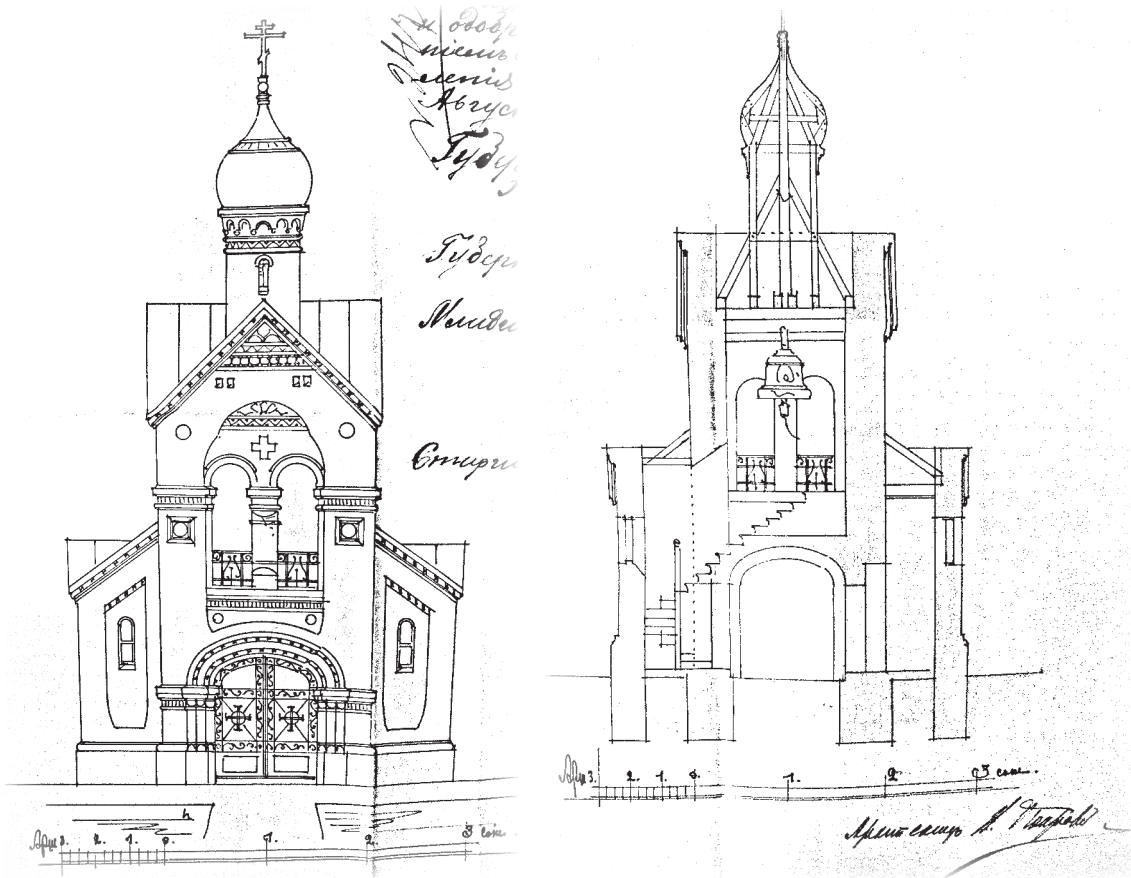
Проект колокольни при Покровской церкви в сл. Городище
