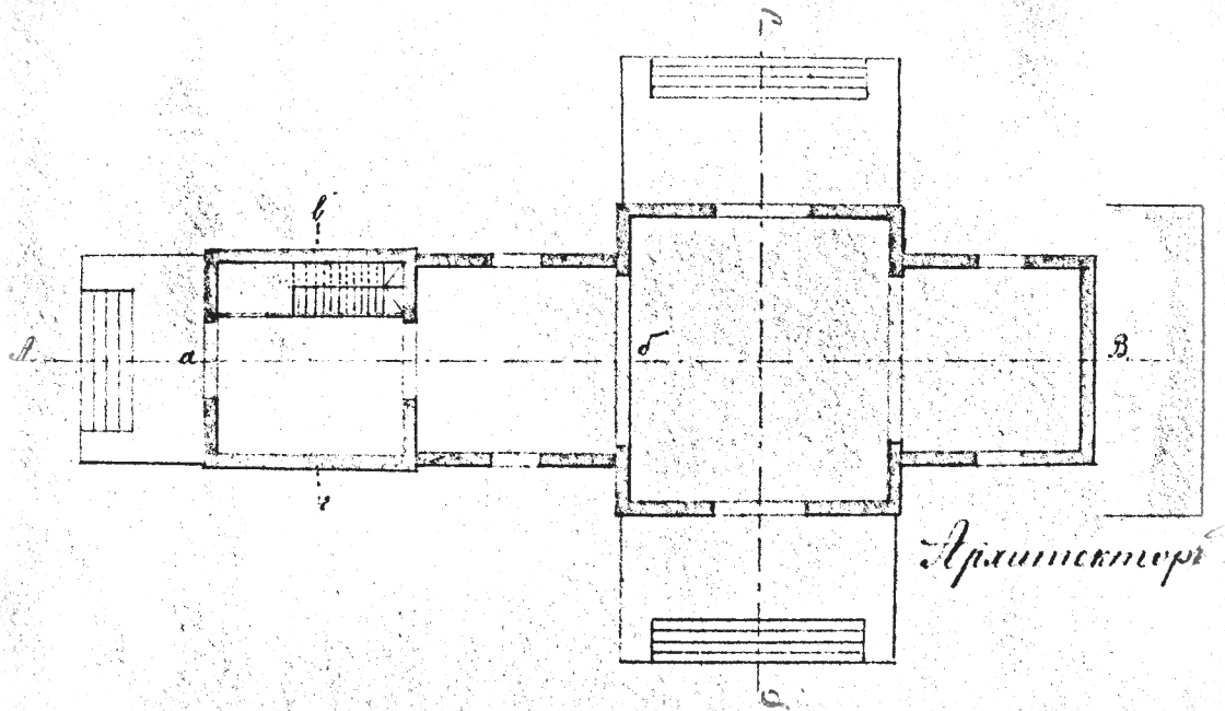
Проект пристройки колокольни к Вознесенской церкви сл. Ново-Боровская
