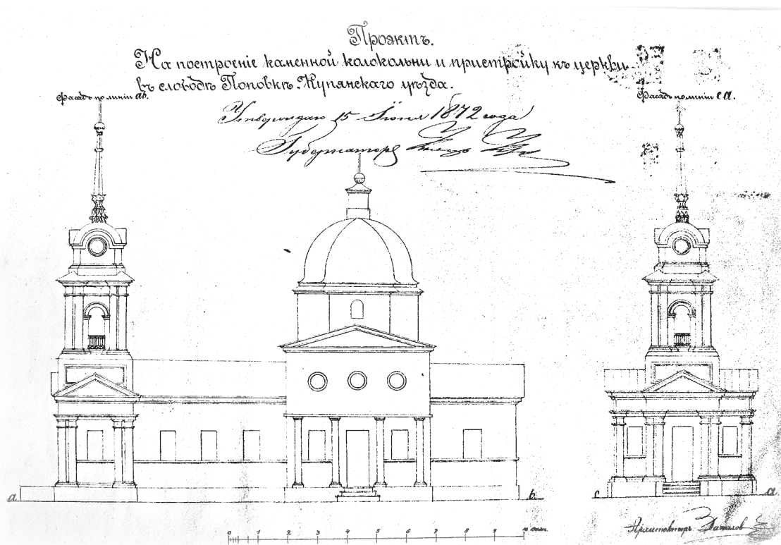
Проект постройки каменной колокольни и пристройки к церкви в сл. Поповке
