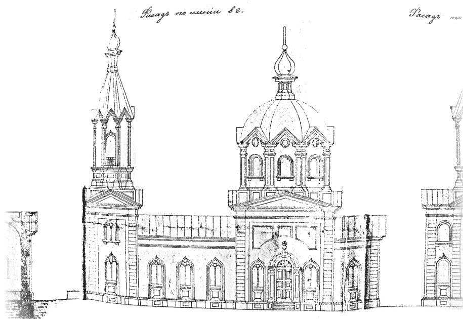
Проект Николаевской церкви в с. Тянюшевка
