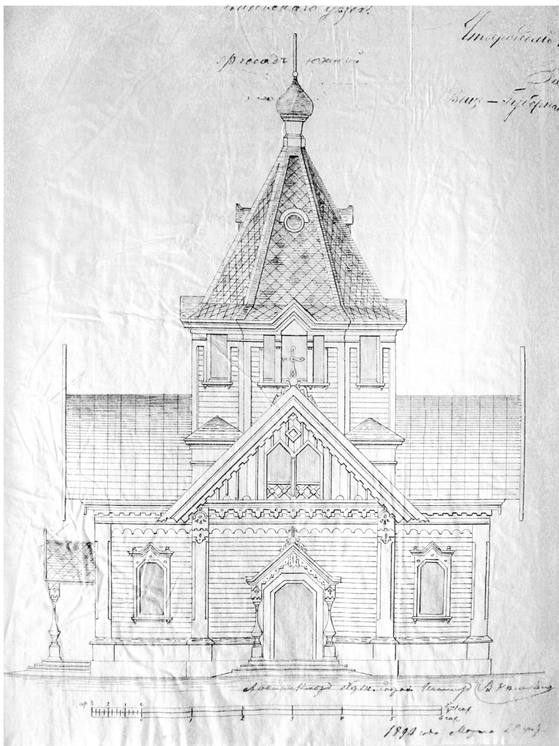
Проект Петропавловской церкви с. Отрада, 1890 г.
